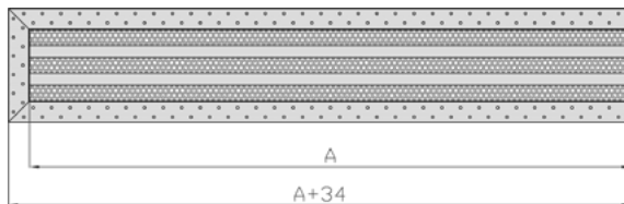
E1 Концевая секция с фланцем
