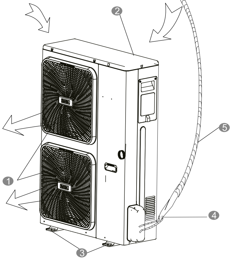
Наружный блок
