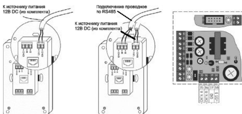
Рис.11 (подключение к источнику питания 12В DC)
